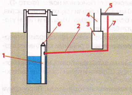
Рис. 1 Схематическое изображение водоснабжения 1 — труба с насосом, 2 — труба отводная, 3 — фундамент дома, 4 — стена, 5 — пол, 6 — пробка, 7 — электрический кабель
