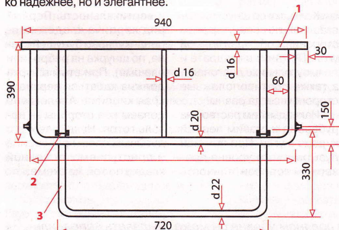
Рис. 1 Чертеж горизонтальной рамы (сиденья) 1 — ось, 2 — шарниры, 3 — П-образная труба (опора)
