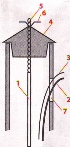
Рис. 2 «Головка» трубы 1 — шнур подвески, 2 — шланг, 3 — электрокабель, 4 — пробка, 5 — цепочка с узелками, 6 — стопор, 7 — «окно» в трубе
