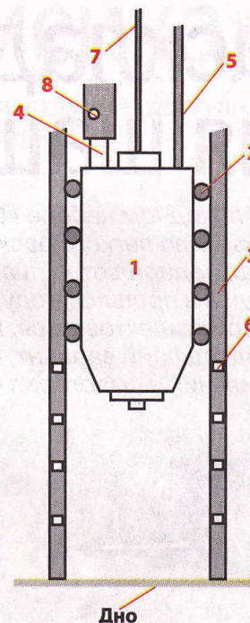
Рис. 3 Расположение насоса в трубе
